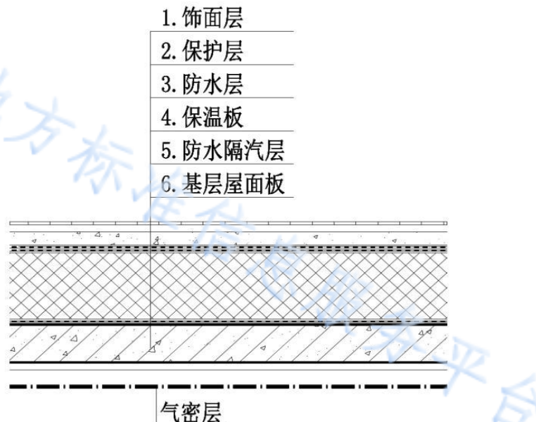
图 3 屋面保温构造做法
